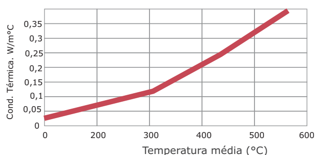
Teste de condutividade térmica x temperatura média
